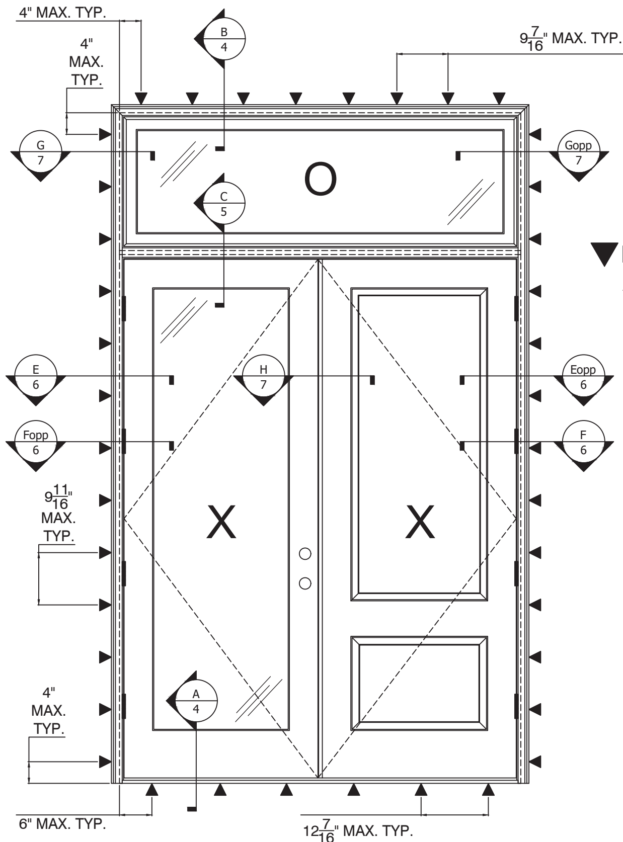
O/XX EXTERIOR VIEW
